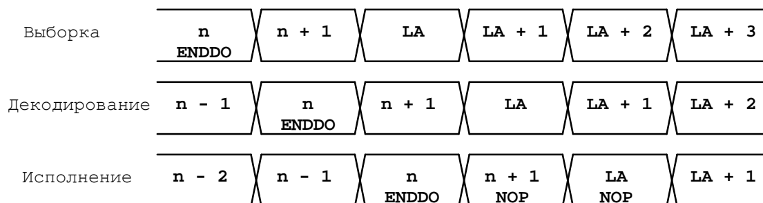
Рисунок 8.6 Работа программного конвейера при выполнении команды ENDDO
