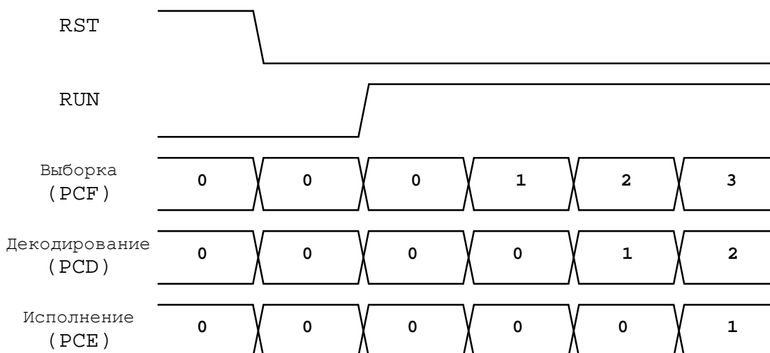
Рисунок 8.3 Работа программного конвейера после начальной установки
