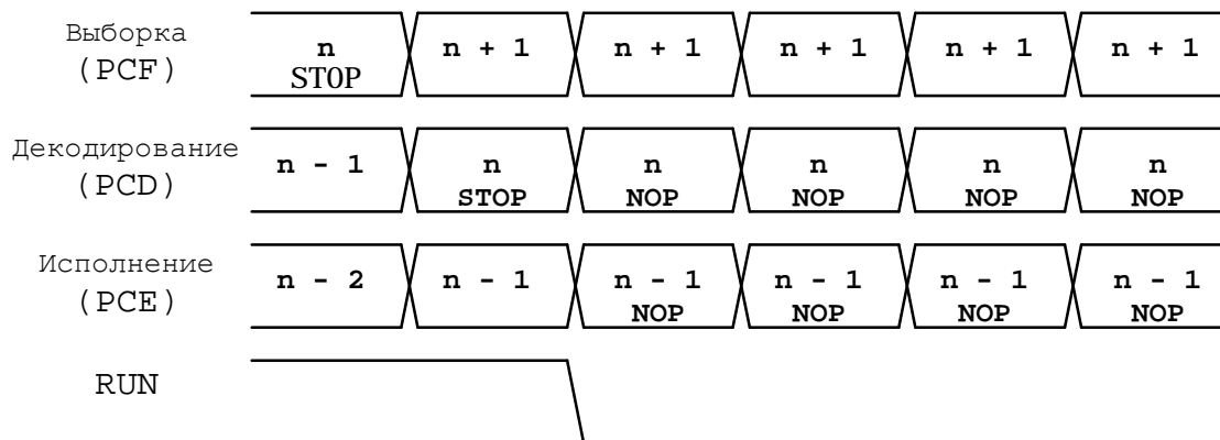
Рисунок 8.9 Работа программного конвейера при исполнении команды STOP
