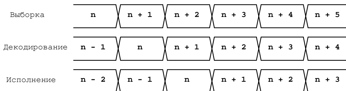
Рисунок 8.1 Работа программного конвейера при последовательной выборке команд
