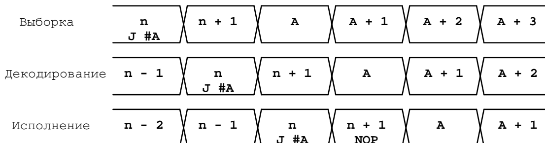
Рисунок 8.4 Работа программного конвейера при программных переходах (команды B, BS, J, JS, RTS).
