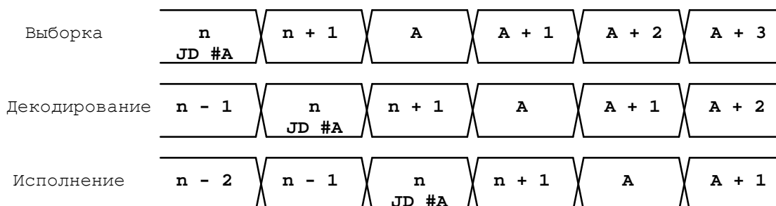
Рисунок 8.5 Работа программного конвейера при отложенных программных переходах (команды BD, JD).
