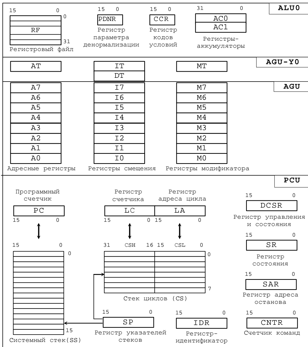
Рисунок 2.1 Программно-доступные регистры DSP-ядра ELcore-14
