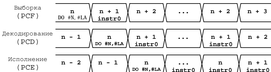
Рисунок 8.8 Работа программного конвейера при выполнении циклов, состоящих из одной инструкции.
