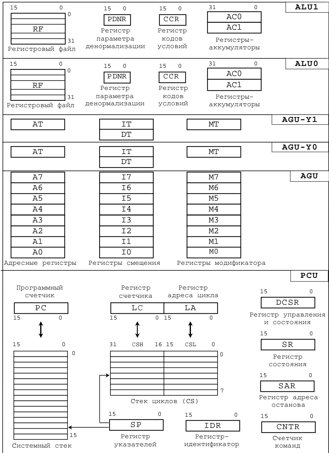
Рис.2.2 Программно-доступные регистры DSP-ядра ELcore-24
