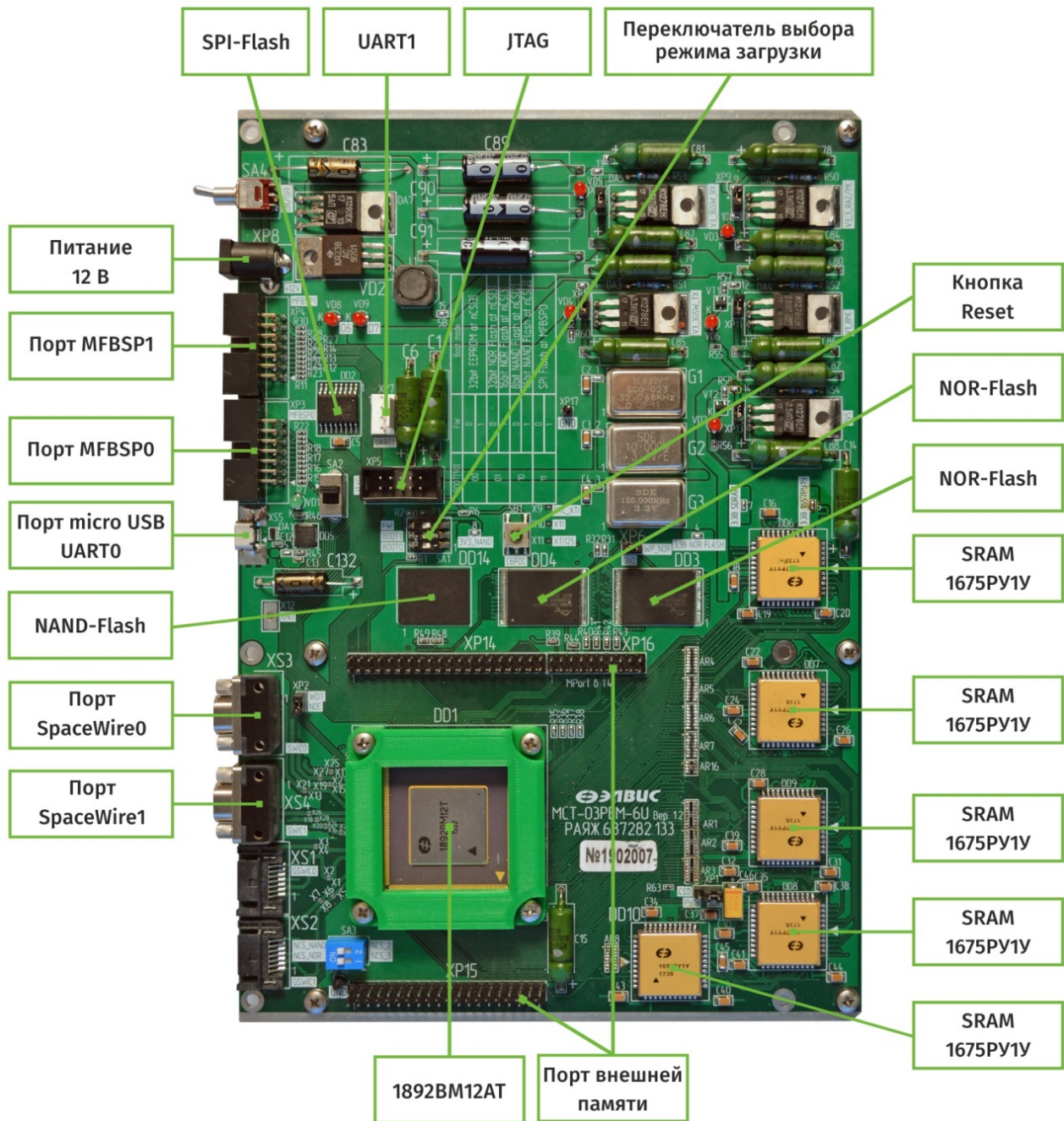
Рисунок 2.3. Внешний вид модуля и его интерфейсы. Лицевая сторона
