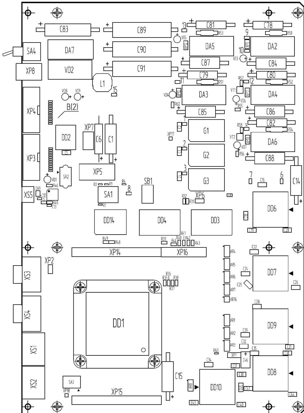
Рисунок 2.1. Расположение элементов на отладочном модуле МСТ-03РЕМ-6U. Лицевая сторона платы
